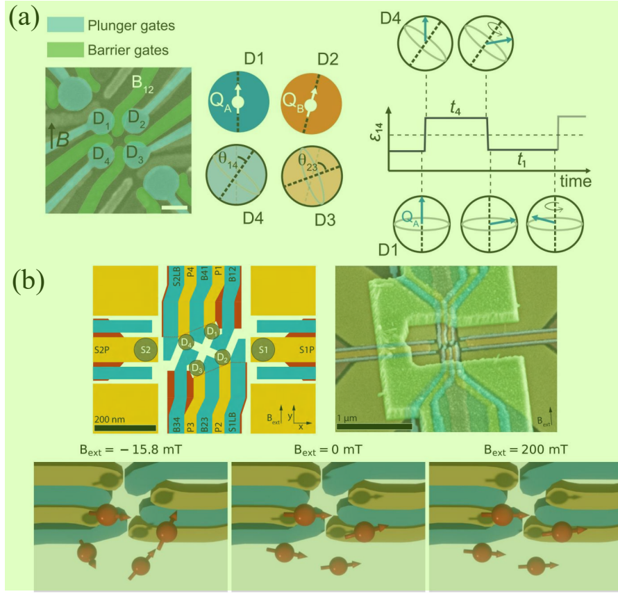
图 3.1 自旋量子比特跳跃门的结构与方案原理
