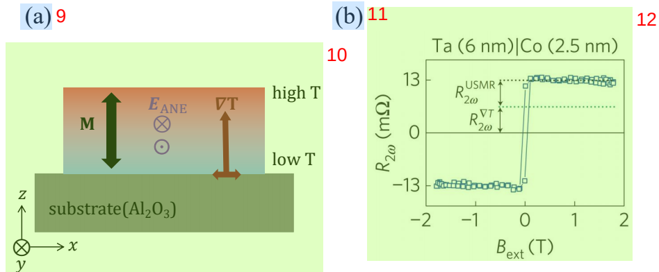
图 5.6 反常能斯特效应示意图 13
