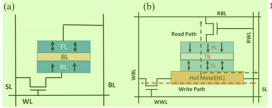
图 2.7 器件写入方式的对比 2
