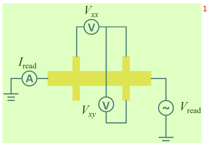
图 5.2 输运测量 SOT 器件的线路结构
