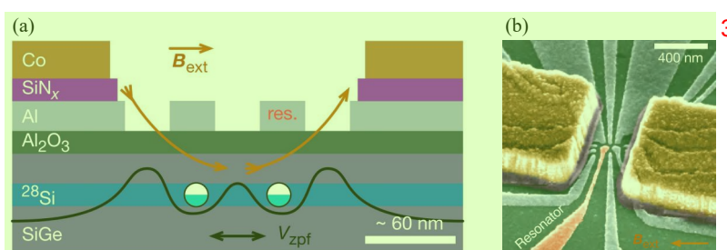
图 1.1 硅基量子器件中的微磁体
