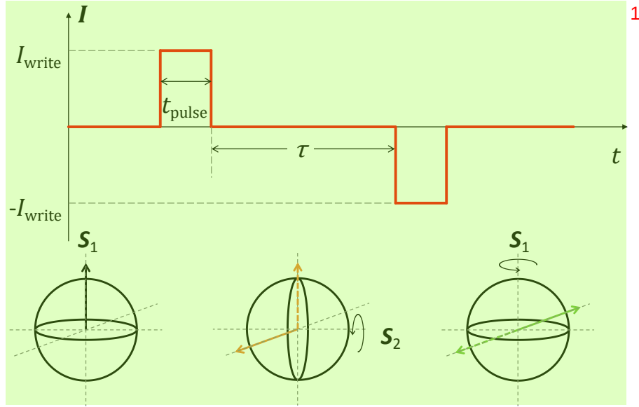
图 3.4 对称设置磁体时的磁场夹角与演化示意图
