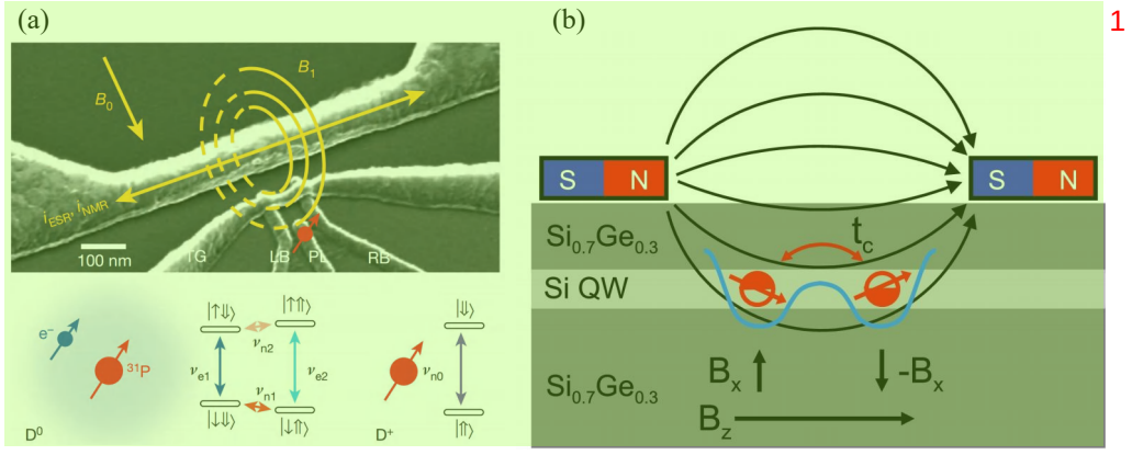
图 2.6 ESR 与 EDSR 示意图 2
