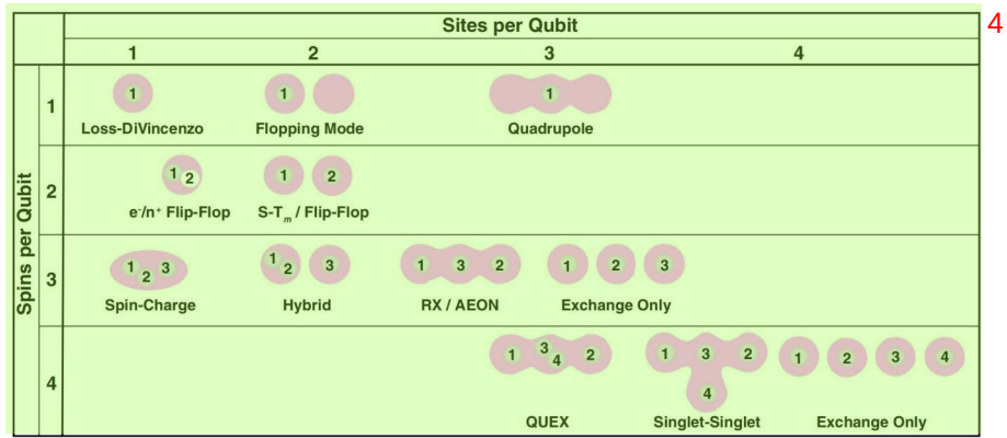
图 2.5 按每个量子比特所含自旋和量子点数量分类的各种自旋量子比特
