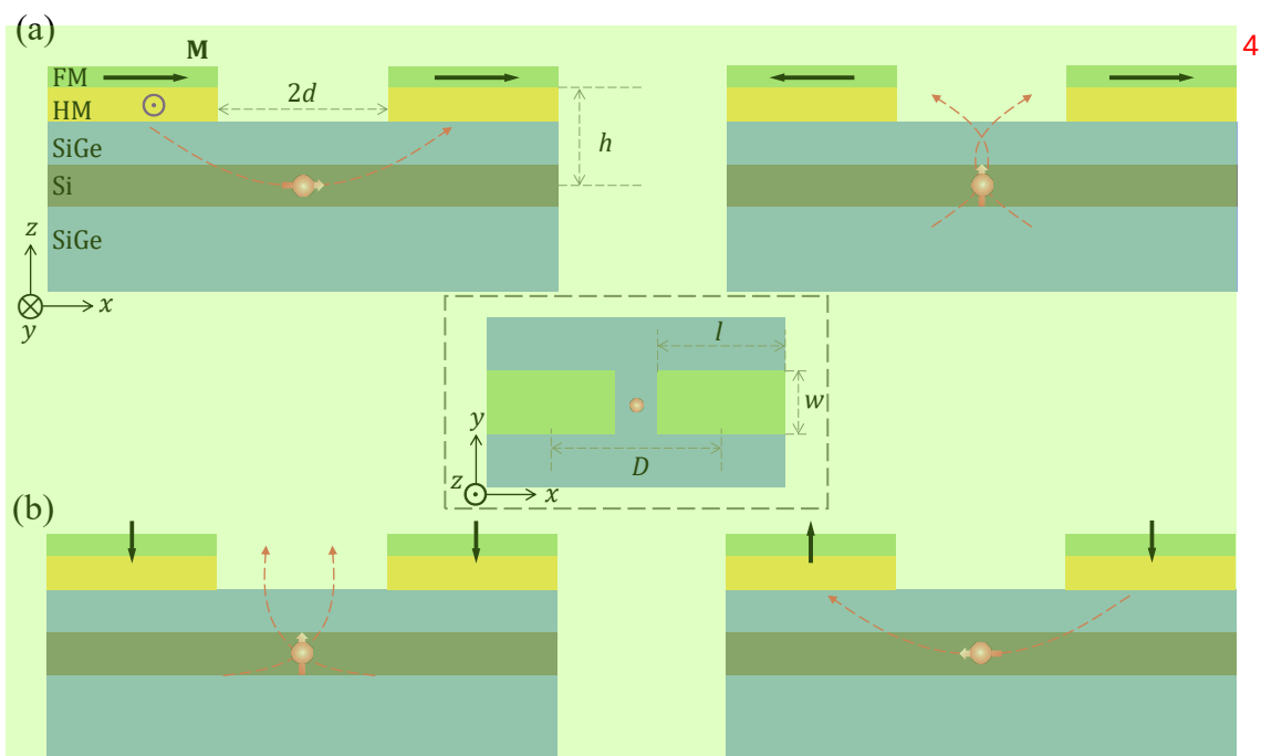
图 3.3 对称设置的不同构型的 SOT 器件产生的磁场示意图 5
