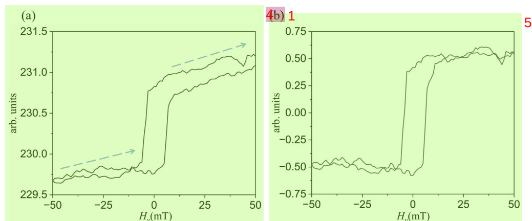
图 4.3 MOKE 测试结果及数据处理后的对比 6
