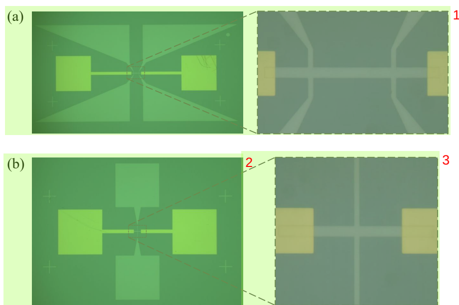
图 4.6 用于测试的 SOT 器件光学照片 4
