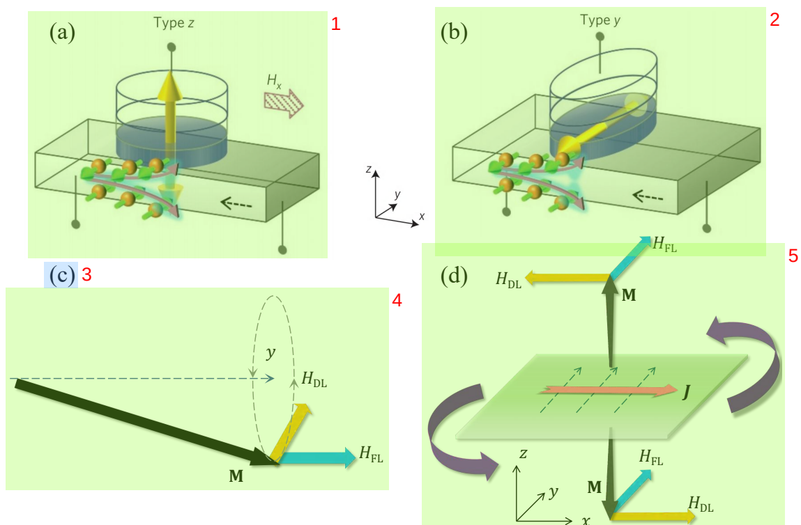
图 2.9 SOT 器件的结构类型与力矩对称性 6
