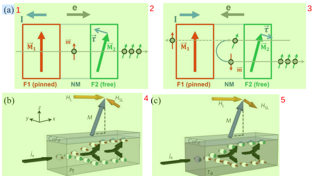
图 2.8 STT 与 SOT 原理示意图 6
