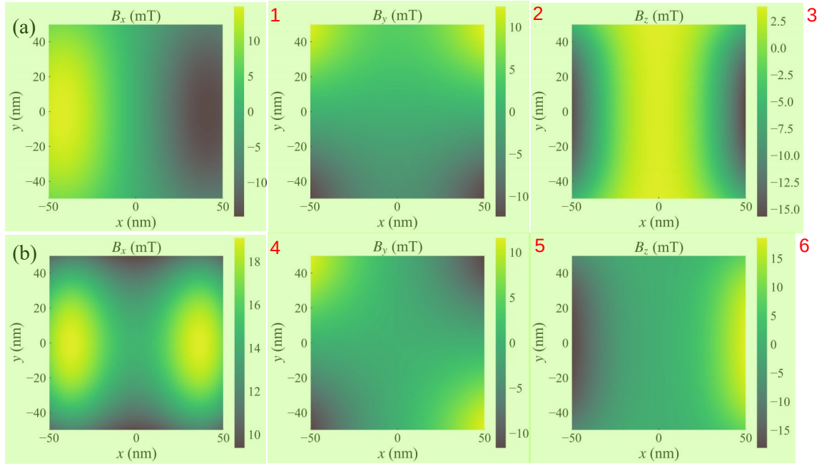
图 3.6 面外 SOT 器件切换前后，磁场在比特周围的分布 7
