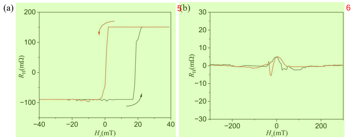
图 5.3 面外磁化构型的 SOT 器件磁性测试结果
