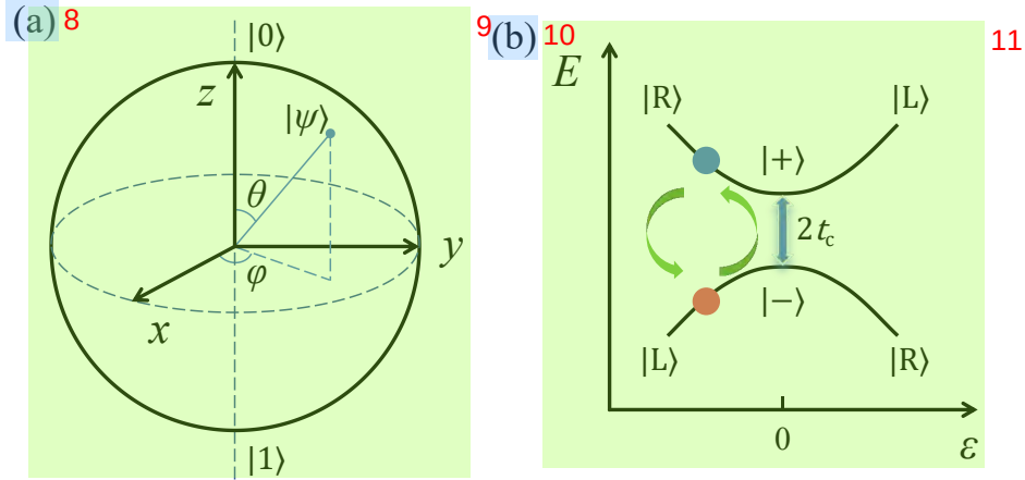
图 2.4 布洛赫球与电荷量子比特能级结构 12
